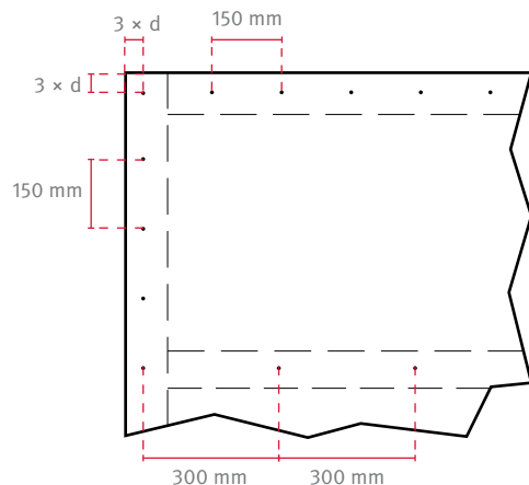
Doporučení pro maximální vzdálenosti spojovacích prostředků u nenosných konstrukcí
